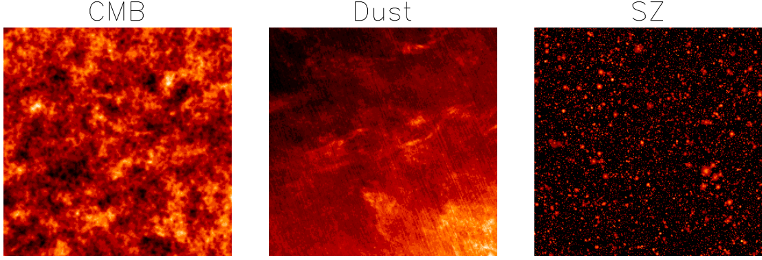
FIG. V.1: Distributions spatiales typiques du CMB, dust et SZ utilisées dans les simulations de ce chapitre. La distribution du SZ est présentée en échelle logarithmique.
